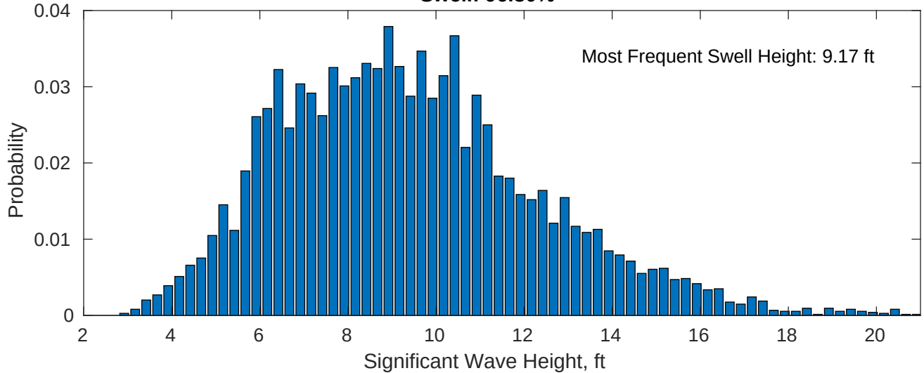
Swell: 96.80%
