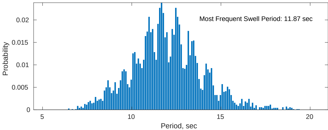
Swell: 81.21%
