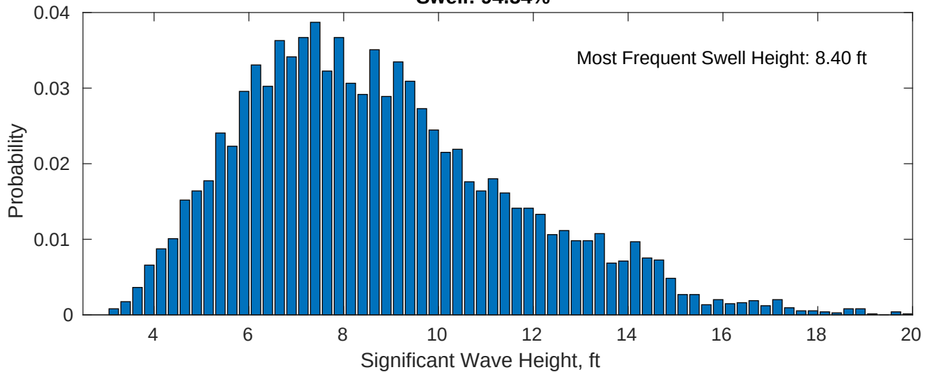
Swell: 94.54%
