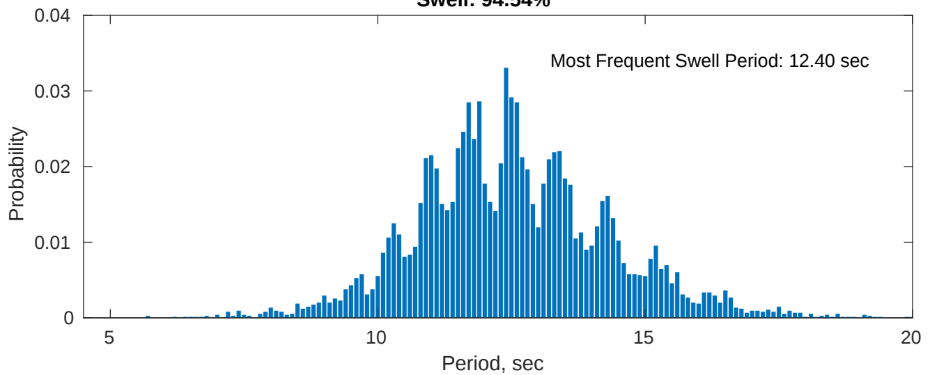
Swell: 94.54%
