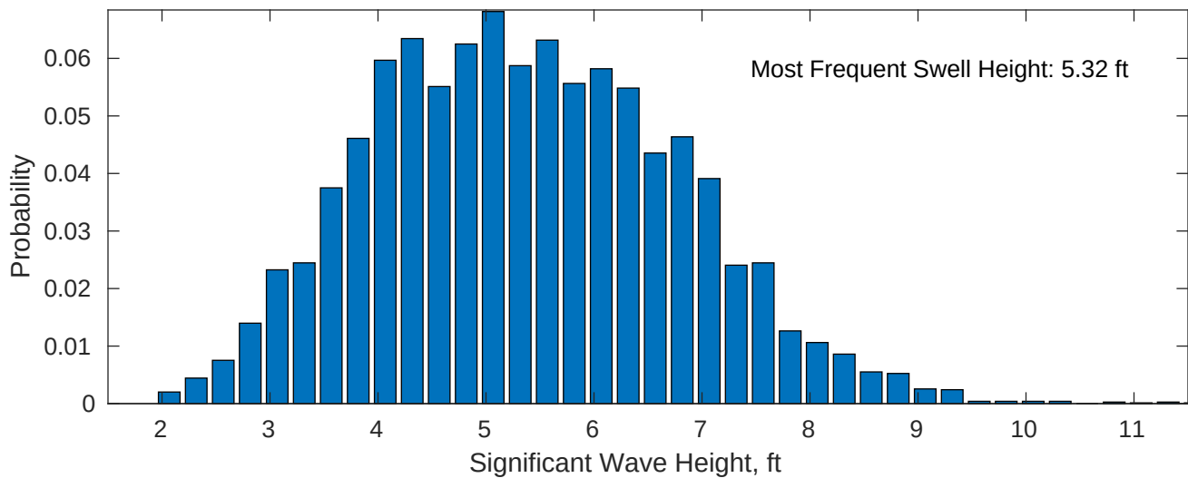
Swell: 98.63%
