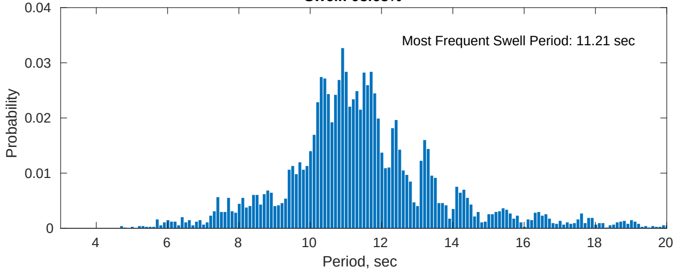
Swell: 98.63%
