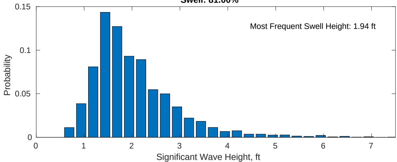
Swell: 81.00%
