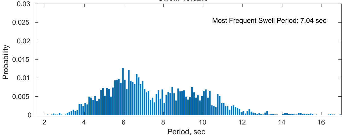
Swell: 49.02%
